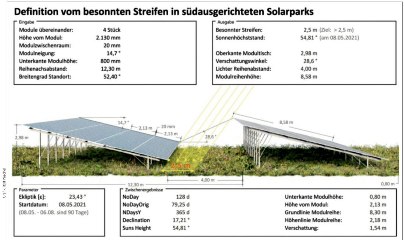
Abb. 8: Berechnung eines besonnten Streifens in südusgerichteten Solarparks. Bild: erstellt von Hauke Nissen für Solpeg und Wattmanufaktur, weitere Infos unter https://www.pvsyst.com/help/solar_geometry.htm
